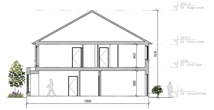
③ H05 Section 1 : 200
